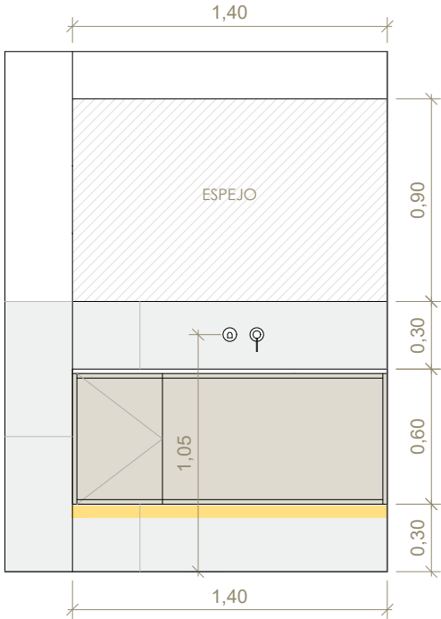
Alzado b-b'
