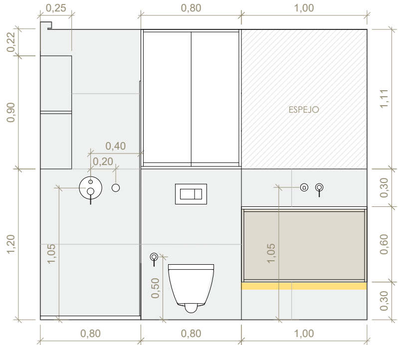
Alzado a-a'
