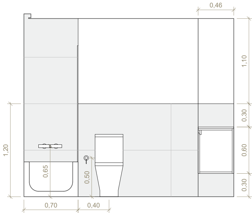
Alzado a-a'
